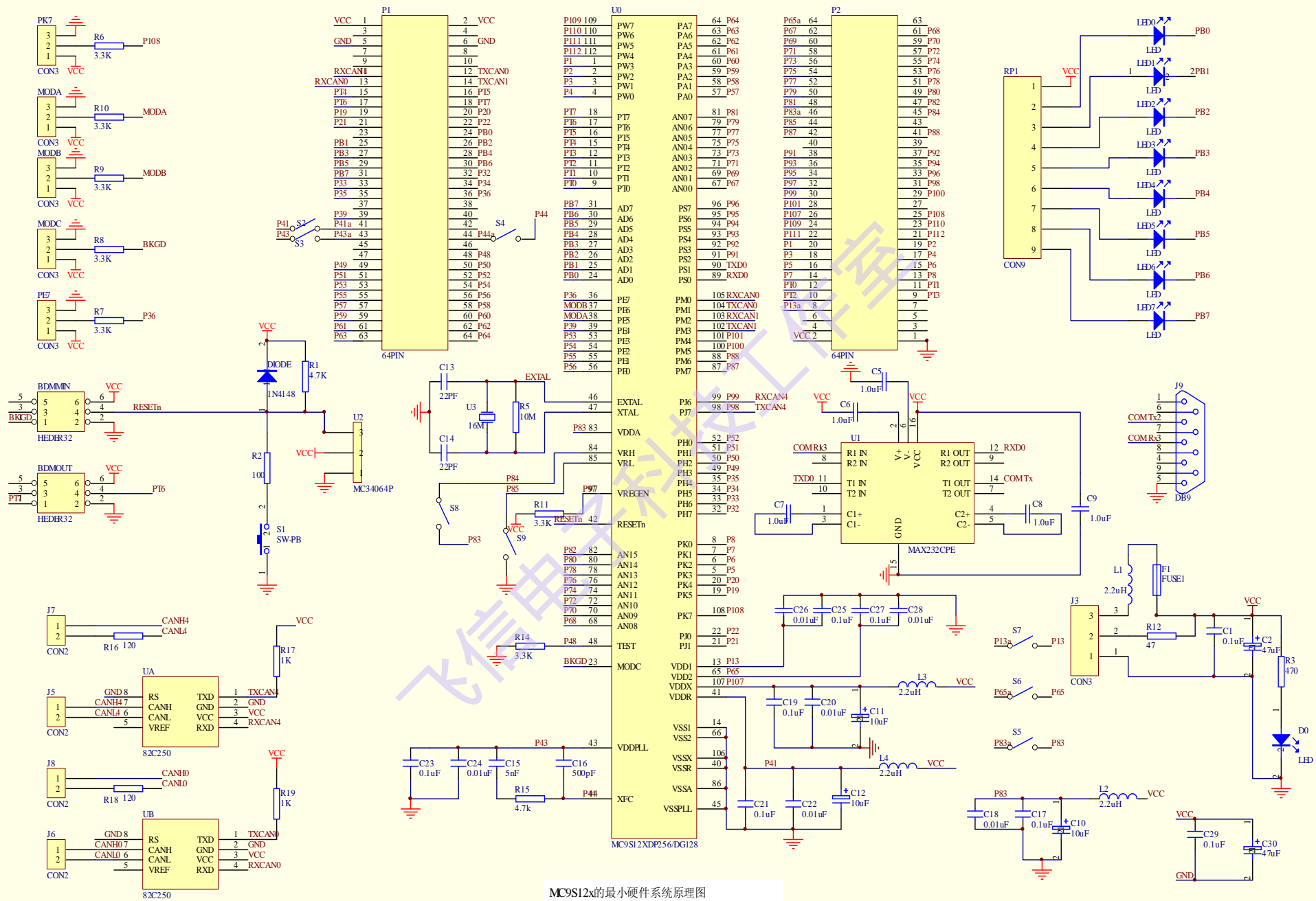
MC9S12x的最小硬件系统原理图
